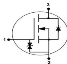
PG-SOT23
